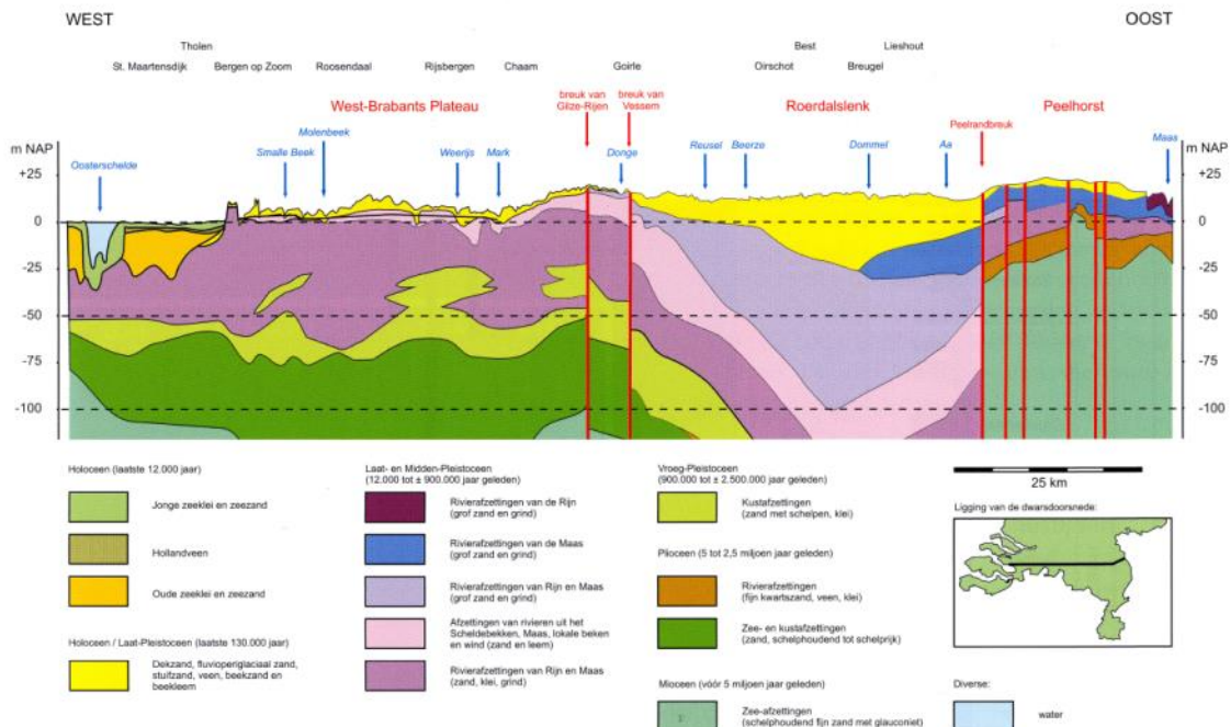
13. Geologische doorsnede van Noord-Brabant. Op de stijgende Peelhorst (uiterst rechts) komen oude zee-afzettingen vrij dicht onder het oppervlak voor. In de dalende Roerdalslenk liggen ze meer dan 300 meter diep; ze kunnen niet weergegeven worden op het profiel, dat slechts tot 100 meter beneden NAP reikt. In de slenk komen bovenaan dikke pakketten relatief jonge dekzand-, beekzand- en rivierafzettingen voor, die dan weer veel dunner zijn of ontbreken op de Peelhorst en op het West-Brabants Plateau (links van de breuk van Gilze-Rijen). Ze zijn in die stijgende gebieden door erosie verdwenen, of werden er nooit afgezet door de hogere ligging. Uiterst links in het profiel, bij de grens met de provincie Zeeland, zijn de diepe insnijdingen te zien van jonge getijdengoulen en van de Oosterschelde.
